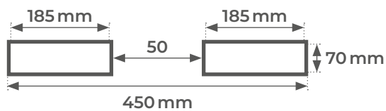
DGG1 PINCE UN FÛT
