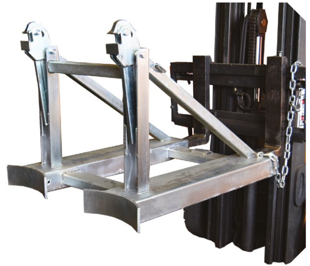
DGG2 PINCE DEUX FÛTS
