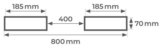
DGG2 PINCE DEUX FÛTS
