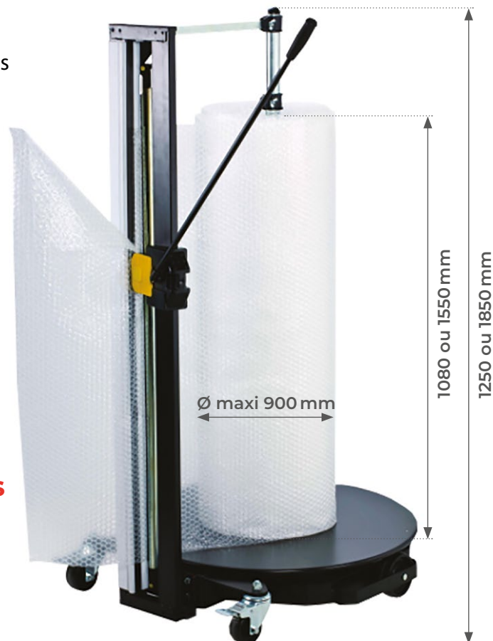
DCV VERTICAL SUR ROULETTES
